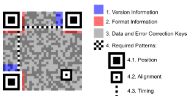
Figura 13: Padrão da imagem do QRCode – Fonte: Wikipédia
